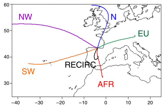
Figura 3. Tipología de las retrotrayectorias y origen. AFR: Norte de África y zona mediterránea de la península; EU: Cantábrico francés; N: Islas Británicas; NW Noratlántico; RECIRC: recirculación a nivel peninsular; SW: Sudatlántico portugués.
