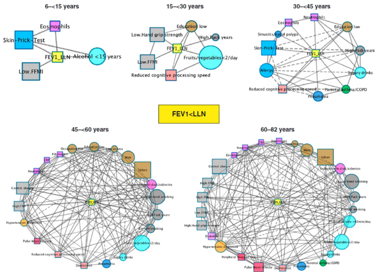
Figura 1. Redes de correlación entre diversos factores (FEV1 inferior al límite inferior de la normalidad (LLN) – cuadrado amarillo en el centro de la red) en diferentes franjas etarias en la cohorte LEAD (Austria). El tamaño de cada nodo es proporcional a su prevalencia en LEAD en esa franja de edad determinada. El color del nodo indica el tipo de variable. Las conexiones entre nodos indican la existencia de correlaciones significativas ( p < 0,05 ) entre ellos y el tipo de línea indica si el OR es superior (continua) o inferior a 1 (discontinua). Figura reproducida de Breyer Kohansal, et al. 4 , con permiso de Am J Respir Crit Care Med.
