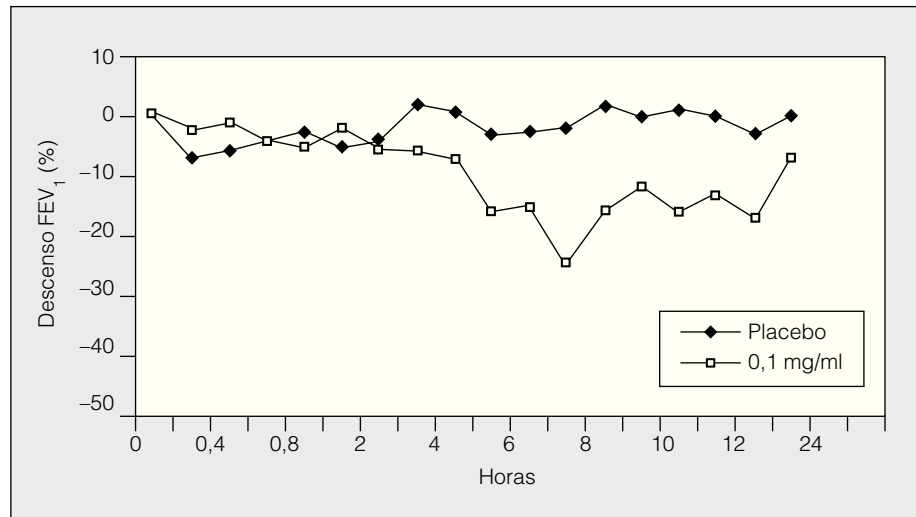
Fig. 1. Prueba de provocación bronquial específica a níquel. Se observa una respuesta positiva tardía, con un descenso máximo del volumen espiratorio forzado en el primer segundo (FEV 1 ) de un 25% a las 8 h de la exposición a 0,1 mg/ml de cloruro de níquel.
